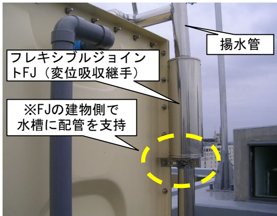
写真-1 揚水管の支持不具合例
