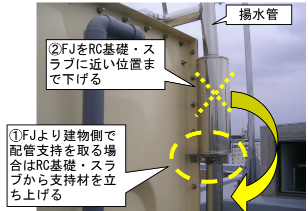
写真-2 揚水管の支持改善例
