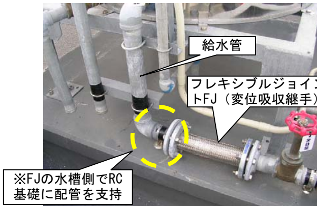
写真-3 給水管の支持不具合例
