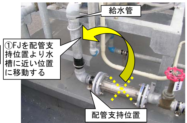
写真-4 給水管の支持改善例
