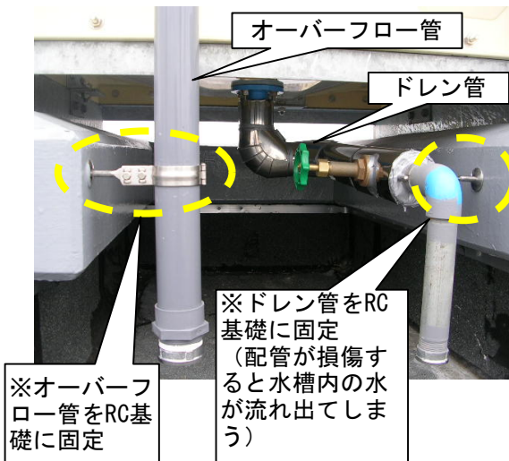
写真-5 ドレン管等の支持不具合例
