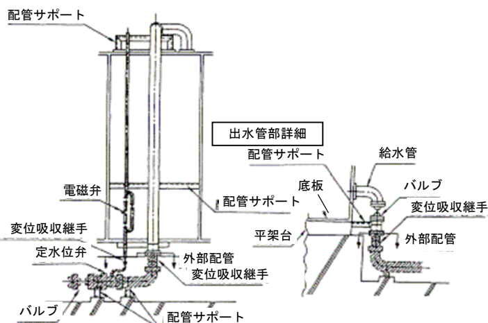
図-3 受水槽（FRP製）の出水管部詳細図 （「建築設備耐震設計・施工指針2005年版」より）
